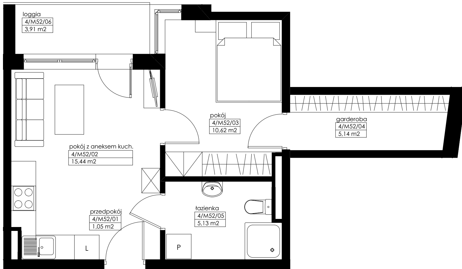
LOKALIZACJA LOKALU MIESZKALNEGO NA RZUCIE KONDYGNACJI RZUT PIĘTRA IV
